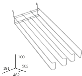
Oddělovač "F", horní, 3 kanály x 57 (pro blister 20 a 28 mm)
