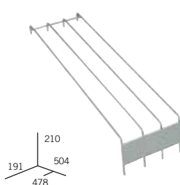
Oddělovač "F", spodní, 3 kanály x 57 (pro blister 20 a 28 mm)
