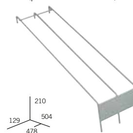
Oddělovač "F", spodní, 2 kanály x 57 (pro blister 20 a 28 mm)
