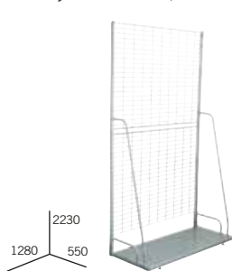
Výstavní vitrina "F", 1280
