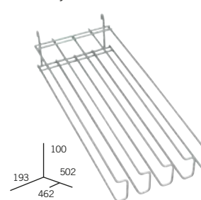
Oddělovač "F", horní, 4 kanály x 42 (Pro tyč 35 a blister 12 mm)
