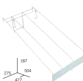
Oddělovač "G", spodní, 3 kanály PJ x 67+85+103
