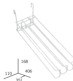
Oddělovač "G", horní, 3 kanály x 30 (pro tyče 12-28 mm)
