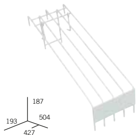
Oddělovač "G", spodní, 4 kanály x 42 (Pro tyč 35 a blister 12 mm)
