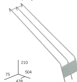
Oddělovač "F", spodní, 2 kanály x 30 (pro tyče 12 - 28 mm)
