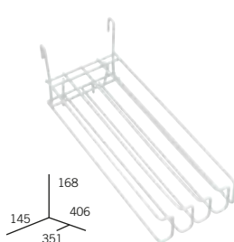
Oddělovač "G", horní, 4 kanály x 30 (pro tyče 12-28 mm)
