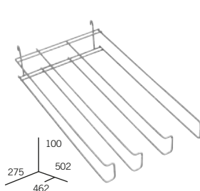
Oddělovač "F", horní, 3 kanály PJ x 67+85+103
