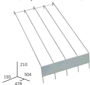
Oddělovač "F", spodní, 4 kanály x 42 (Pro tyč 35 a blister 12 mm)
