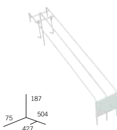
Oddělovač "G", spodní, 2 kanály x 30 (pro tyče 12-28 mm)
