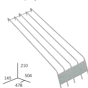
Oddělovač "F", spodní, 4 kanály x 30 (pro tyče 12 - 28 mm)
