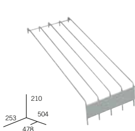
Oddělovač "F", spodní, 4 kanály x 57 (pro blister 20 a 28 mm)
