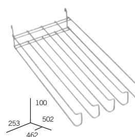
Oddělovač "F", horní, 4 kanály x 57 (pro blister 20 a 28 mm)
