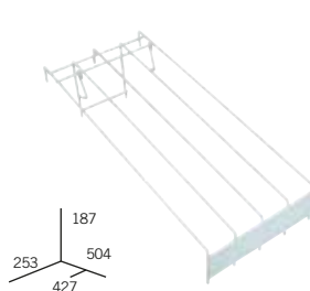
Oddělovač "G", spodní, 4 kanály x 57 (pro blister 20 a 28 mm)
