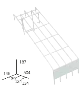
Oddělovač "G", spodní, 16 kanály x 30 (pro tyče 12 mm)
