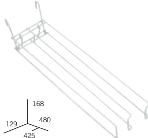
Oddělovač "G", horní, 2 kanály x 57 (pro blister 20 a 28 mm)
