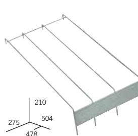
Oddělovač "F", spodní, 3 kanály PJ x 67+85+103
