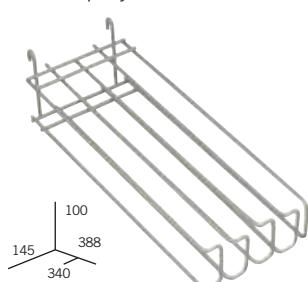
Oddělovač "F", horní, 4 kanály x 30 (pro tyče 12 - 28 mm)
