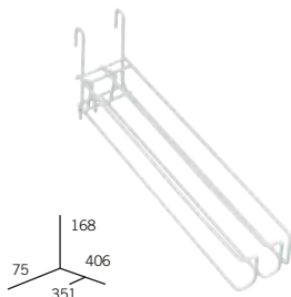
Oddělovač "G", horní, 2 kanály x 30 (pro tyče 12-28 mm)
