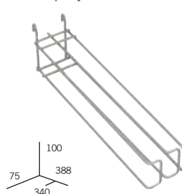
Oddělovač "F", horní, 2 kanály x 30 (pro tyče 12 - 28 mm)
